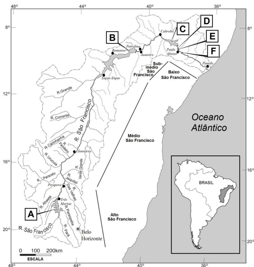
Figura 1. Bacia hidrográfica do rio São Francisco com suas subdivisões: alto, médio, submédio e baixo São Francisco. Reservatórios: Três Marias (A), Sobradinho (B), Itaparica (C), Complexo de Paulo Afonso (D e E) e Xingó (F). Fonte: Sato & Godinho (2003) modificado.
