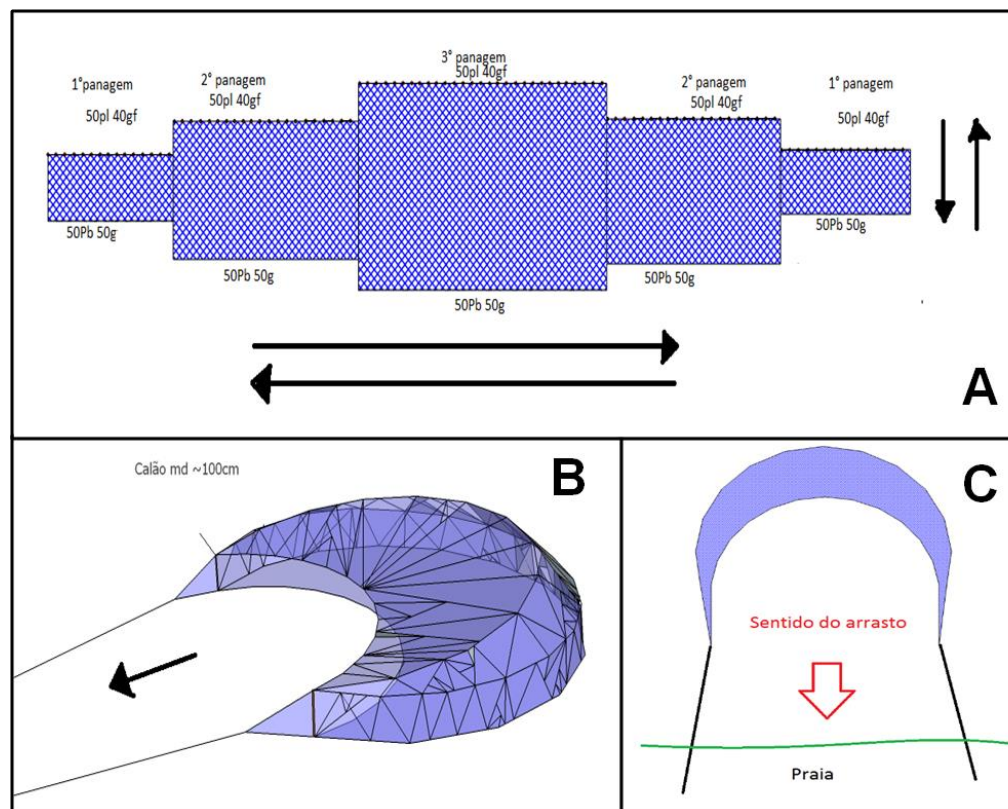
Figura 5: Plano padrão (A) e esquema de funcionamento (B e C) das redes de arrasto de praia tipo “mangote”, utilizadas na pesca de arrasto de praia tipo “mangote” no litoral de Pernambuco (Imagens – Eduardo Rangel) ( ↑ ↓ - altura da rede na panagem, ↔ número de malhas no comprimento, md - madeira.
