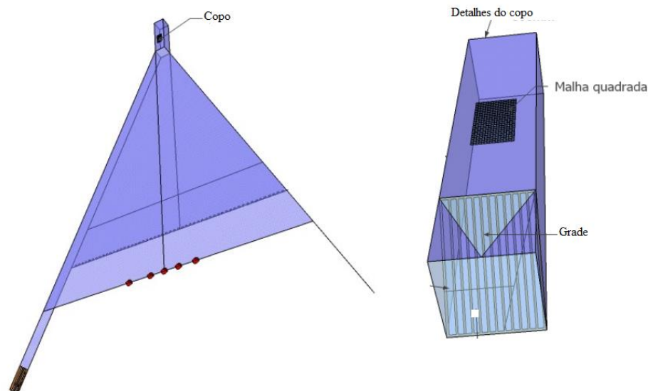
Figura 5 – Esquema de utilização de uma rede de pesca de camarões utilizando a malha quadrada e a grade como DRFA.
