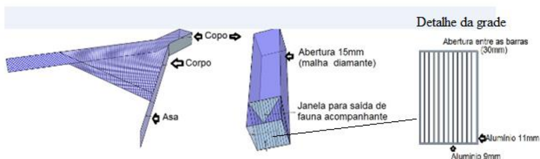
Figura 4 – Esquema de utilização de uma rede de pesca de camarões utilizando a grade como DRFA.
