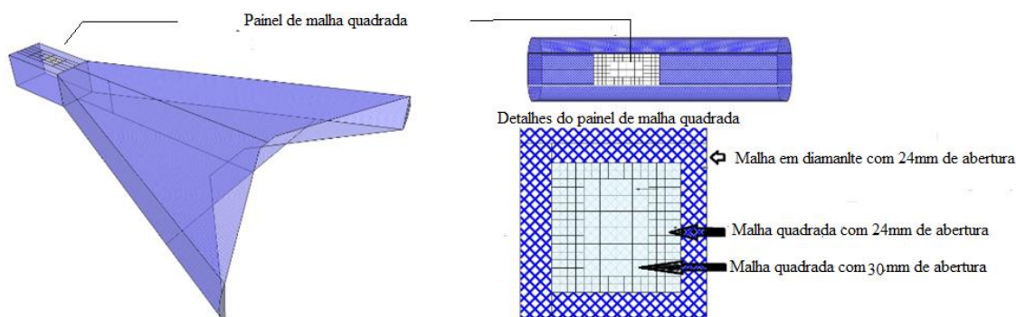
Figura 3 – Esquema de utilização de uma rede de pesca de camarões utilizando a malha quadrada como DRFA.
