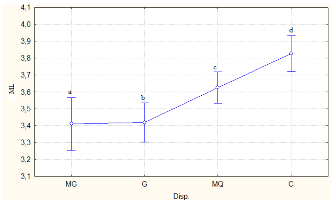
Figura 20 – Larguras de Haemulidae capturados no dispositivo controle (C) e nos três DRFA: grade (G), malha quadrada (MQ) e malha quadrada e grade (MG). As larguras em (a) = (b e c), (a) ≠ (d); (b) < (c) < (d), porém, estatisticamente não existe diferença entre os três dispositivos ao ser analisado com o teste de Post hoc HSD Tukey (ML – maior largura e Disp – dispositivo).
