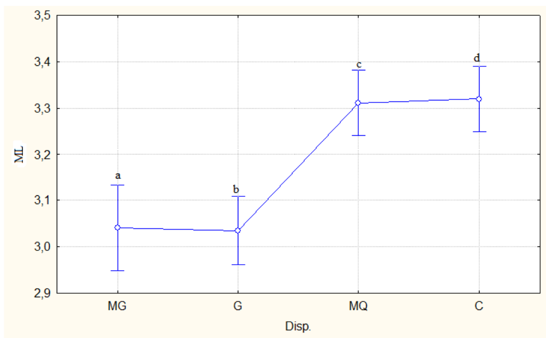
Figura 16 – Larguras de Scianidae capturados no dispositivo controle (C) e nos três DRFA: grade (G), malha quadrada (MQ) e malha quadrada e grade (MG). As larguras em (a) = (b) e (c) = (d), porém (a, b) ≠ (c, d) (ML – maior largura e Disp – dispositivo).
