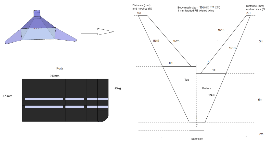
Figura 6 - Detalhes da rede de arrasto de camarão utilizada no litoral sul de Pernambuco e detalhes das portas utilizadas para abertura dessas redes (Imagem - Eduardo Rangel).
