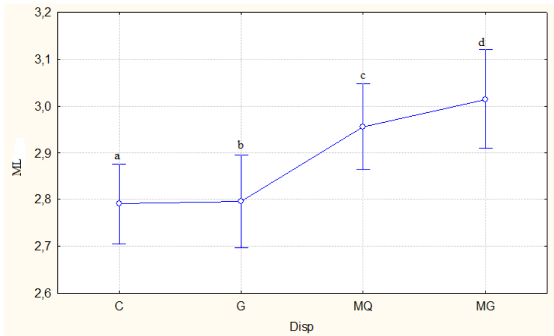
Figura 14 – Larguras de Pristigasteridae capturados no dispositivo controle (C) e nos três DRFA: grade (G), malha quadrada (MQ) e malha quadrada e grade (MG). As larguras em (a) = (b) e (c) = (d), (b) < (c), mesmo que não estatisticamente significativo ao ser analisado com o teste de Post hoc HSD Tukey e (a, b) ≠ (d) (ML – maior largura e Disp – dispositivo).
