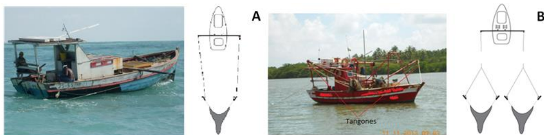
Figura 3- A) Embarcação utilizada na pesca de camarão com arrasto de popa simples, e B) Embarcação utilizada na pesca de camarão com tangones, utilizados no litoral do estado de Pernambuco (foto – Eduardo Rangel).
