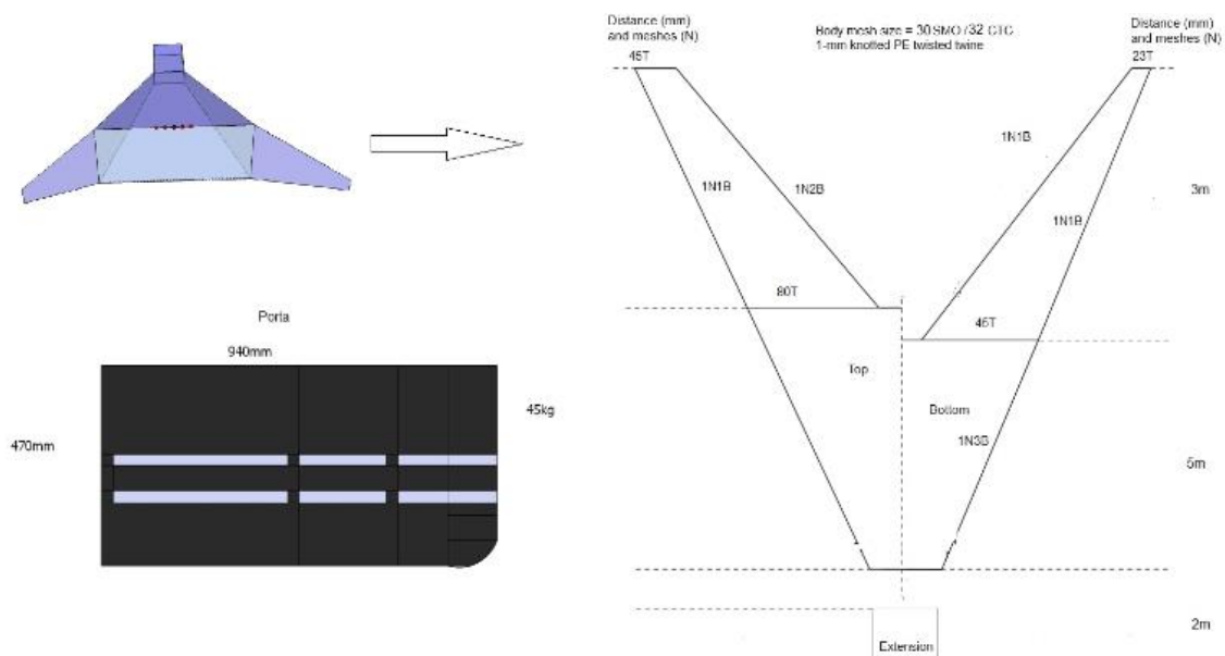
Figura 2 - Detalhes da rede de arrasto de camarão utilizada no litoral sul de Pernambuco e detalhes das portas utilizadas para abertura dessas redes.
