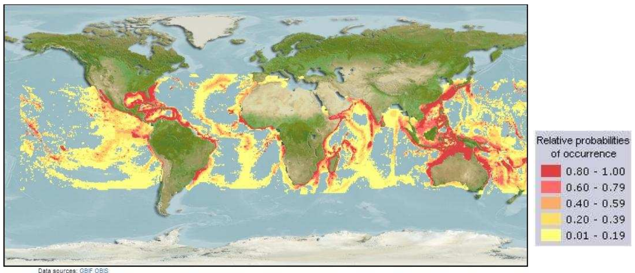
Figura II - Distribuição mundial do tubarão lombo-preto ( Carcharhinus falciformis ). (Fonte: Fishbase e aquamaps.org)
