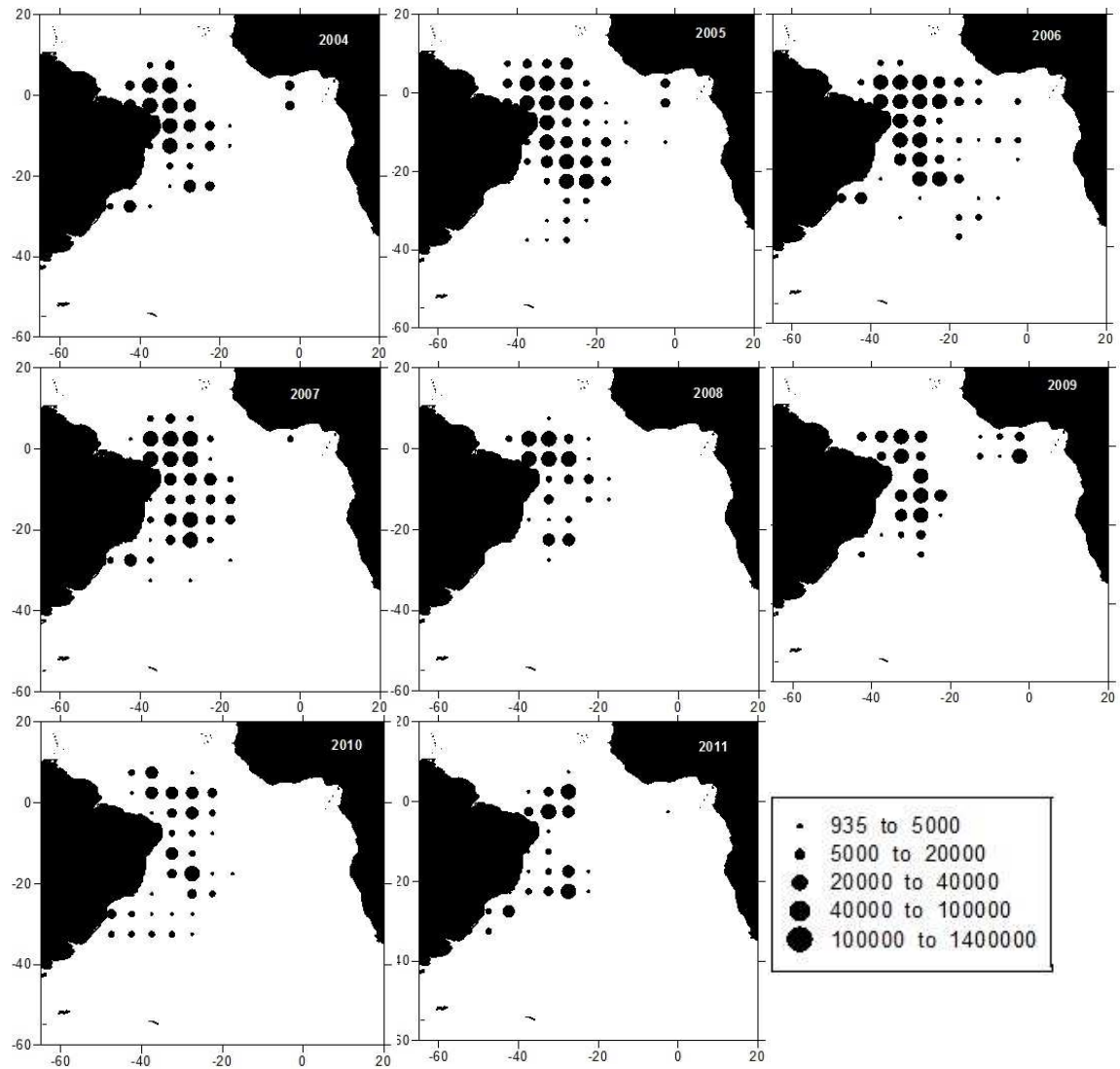
Figura 3- Distribuição espacial anual do esforço de pesca da frota atuneira brasileira arrendada, em quadrados de 5° x 5° de latitude e longitude, de 2004 a 2011, na região Equatorial e Oceano Atlântico Sul Ocidental.
