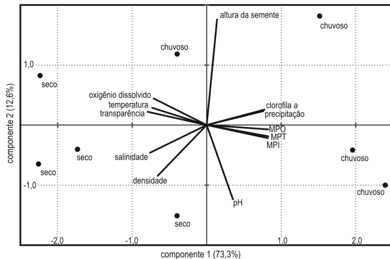
Figura 4. Análise de componentes principais indicando a relação entre as variáveis ambientais e biológicas para as amostragens efetuadas no ponto II.
