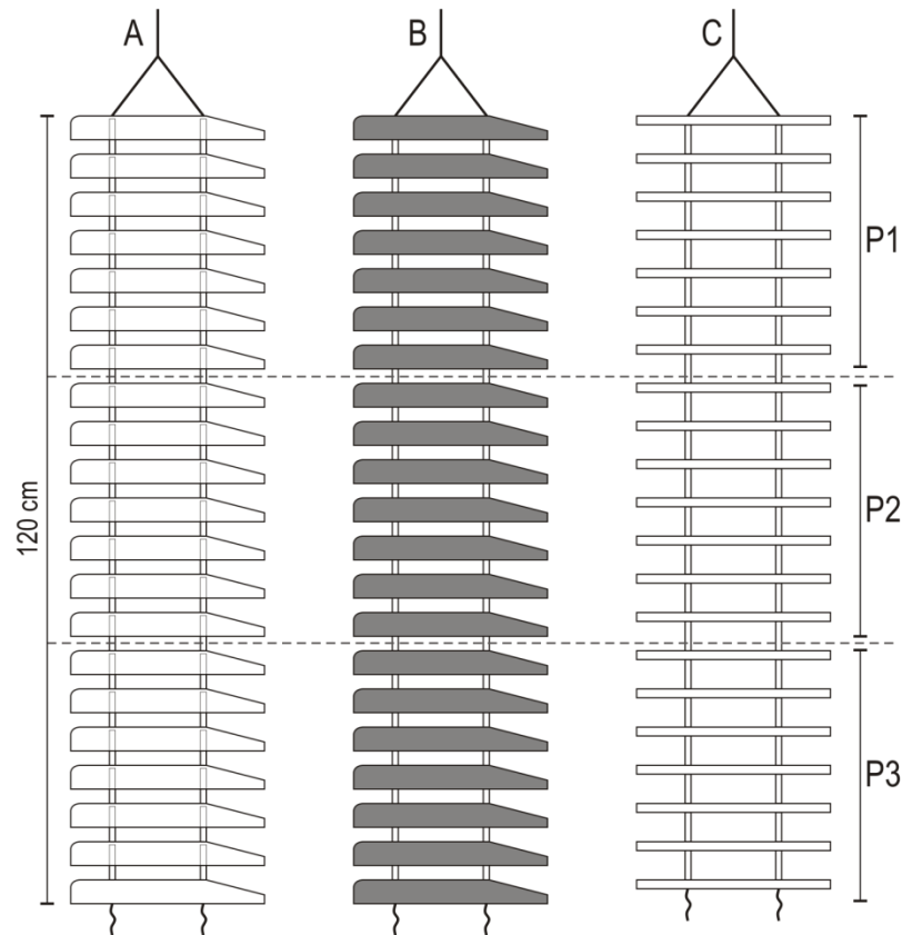
Figura 2. Diagrama esquemático mostrando os três tipos de coletores (A - PET transparente, B - PET verde, C - placa de PVC) e os intervalos de profundidade estudados (P1 0-40 cm, P2 41-80 cm, P3 81-120 cm).
