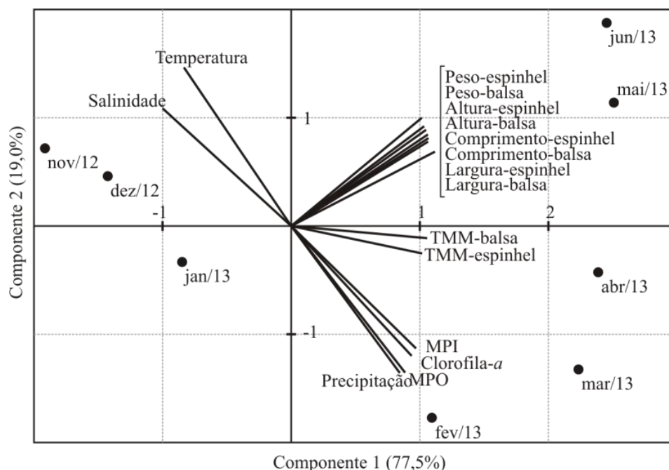
Figura 2. Análise de componentes principais indicando a associação entre as variáveis ambientais (salinidade, temperatura, clorofila a , precipitação e material particulado orgânico e inorgânico) e biológicas (TMM - taxa de mortalidade mensal, peso total, altura, comprimento e largura das valvas) de C. gasar cultivada em sistemas de cultivo flutuante (balsa e espinhel).
