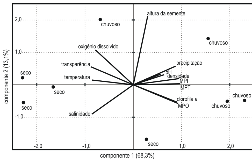
Figura 3. Análise de componentes principais indicando a relação entre as variáveis ambientais e biológicas para as amostragens efetuadas no ponto I.
