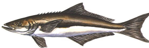
Figura 1 – Exemplar de beijupirá ( Rachycentron canadum ). Fonte: www.fishbase.org.br .
