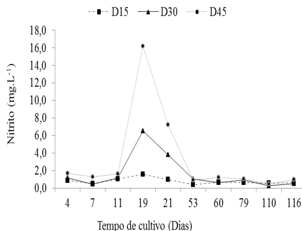
Figura 2. Variações médias dos compostos nitrogenados (A. amônia total, \text{NH}_3+\text{NH}_4 , e B. nitrito, \text{NO}_2 ) durante 128 dias, no cultivo de juvenis de tilápia do Nilo O. niloticus sob diferentes densidades de estocagem com tecnologia de bioflocos
