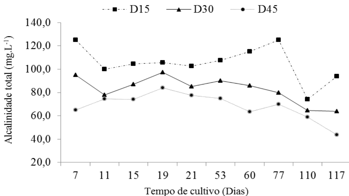
Figura 1. Variações médias de alcalinidade total ( \text{mg.L}^{-1} \text{CaCO}_3 ) durante 128 dias, no cultivo de juvenis de tilápia do Nilo O. niloticus sob diferentes densidades de estocagem com tecnologia de bioflocos
