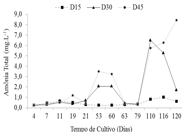
Figura 2. Variações médias dos compostos nitrogenados (A. amônia total, \text{NH}_3+\text{NH}_4 , e B. nitrito, \text{NO}_2 ) durante 128 dias, no cultivo de juvenis de tilápia do Nilo O. niloticus sob diferentes densidades de estocagem com tecnologia de bioflocos
