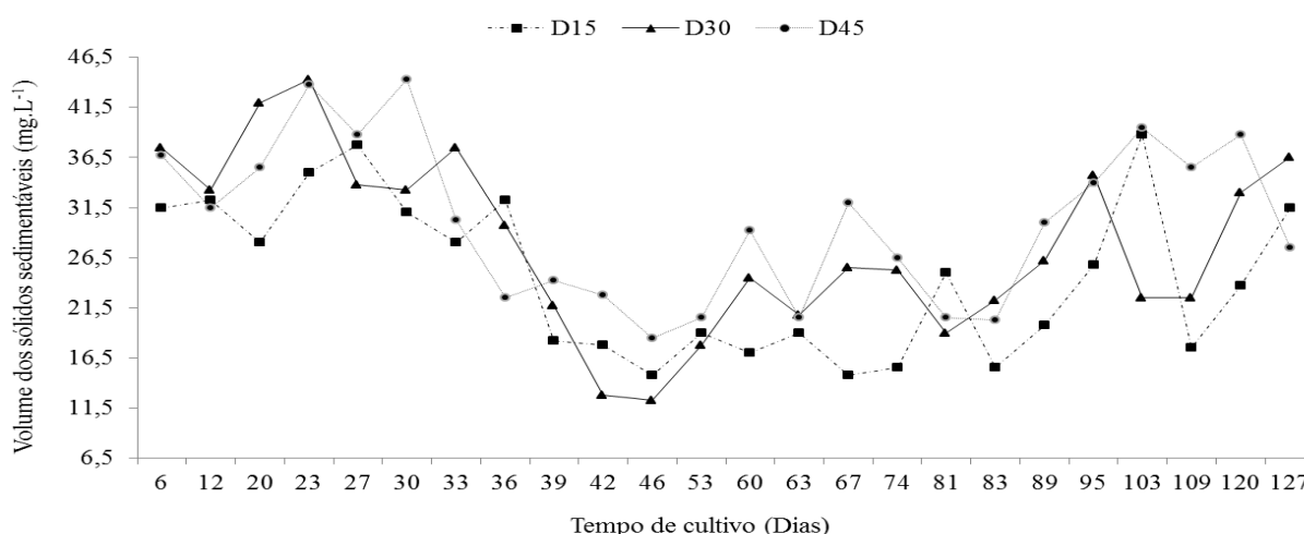
Figura 3. Volume médio dos sólidos sedimentáveis durante 128 dias, no cultivo de juvenis de tilápia do Nilo O. niloticus sob diferentes densidades de estocagem com tecnologia de bioflocos
