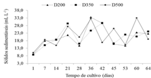
Figura 1. Variações físico-químicas da água no cultivo de tilápia do Nilo O. niloticus , na fase de alevinagem, sob as diferentes densidades de estocagem em sistema de bioflocos.
